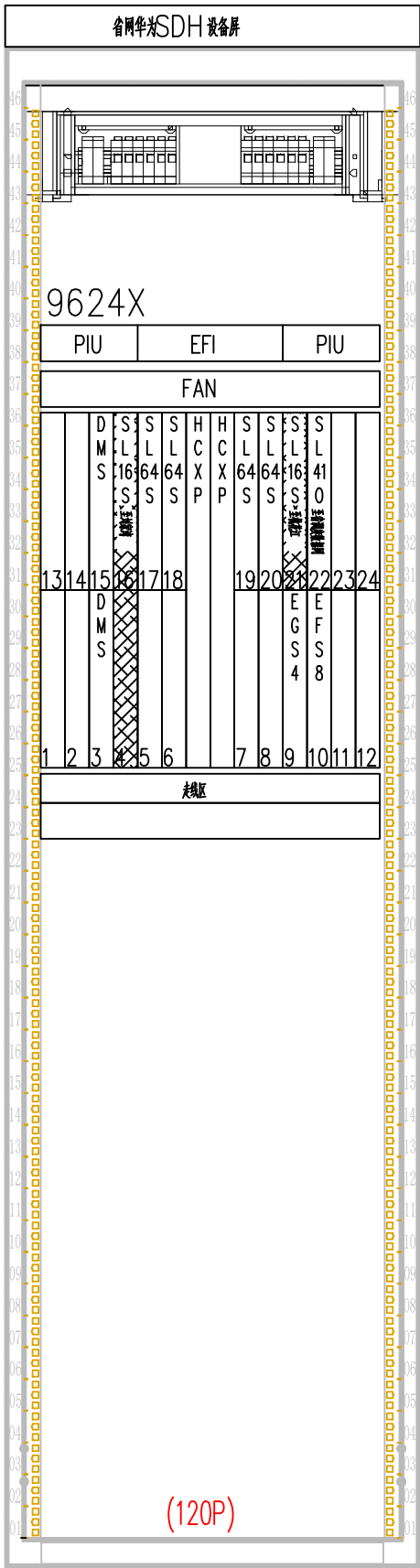
省网A1平面SDH设备机架图
