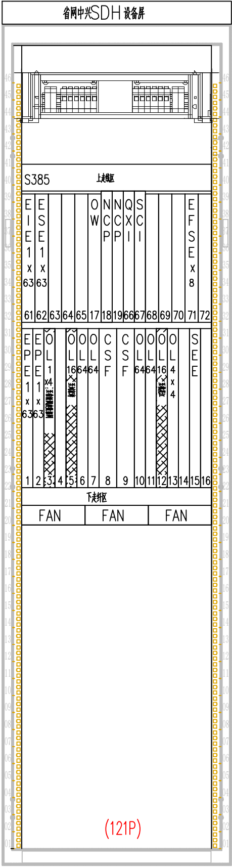
省网A2平面SDH设备机架图
